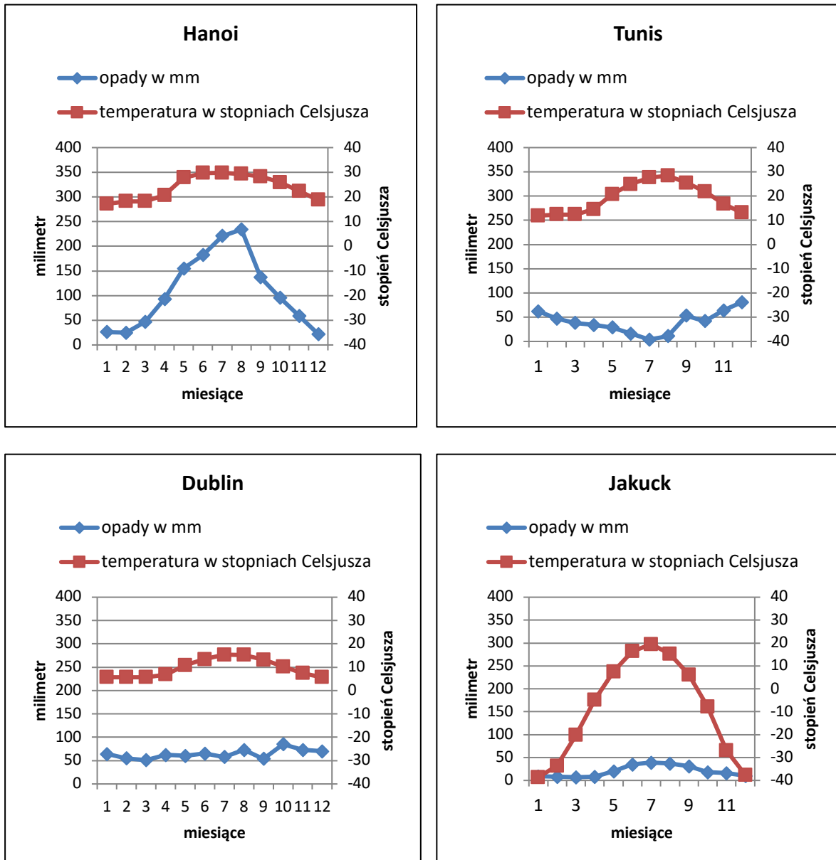
Figura 1. Diagramy klimatyczne składają się z diagramu opadów i diagramu temperatury. Opady odczytuje się po lewej stronie w milimetrach, temperaturę po prawej stronie w stopniach Celsjusza. Diagramy przedstawiają średnie opady i temperaturę od stycznia do grudnia.
